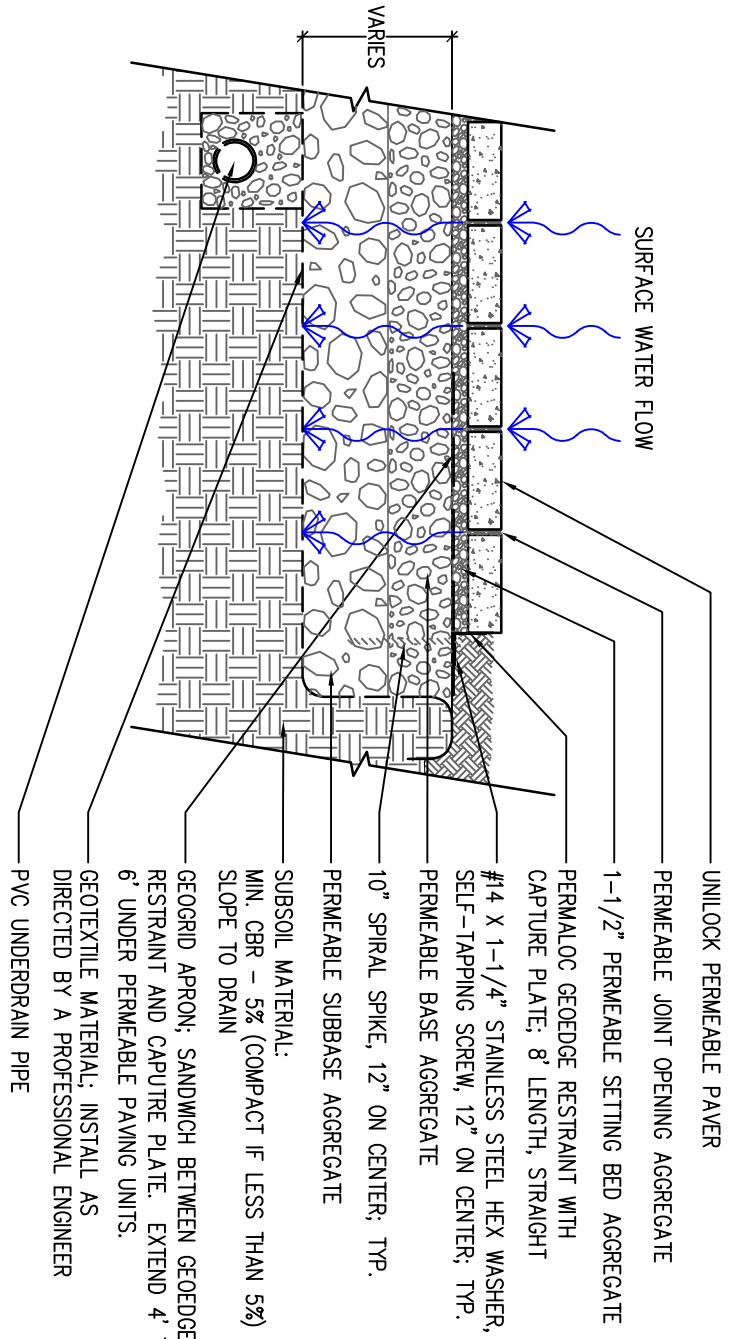
8 Permeable Pavers with Aluminum Edge Restraint CS-COM-PERM-PERMALOC
