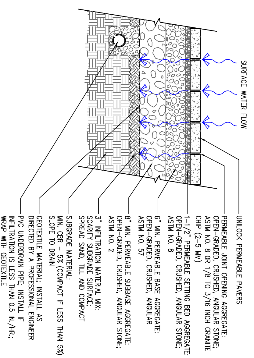
9 LD-Low Infiltration Permeable Paver Section CS-COM-PERM-T3
